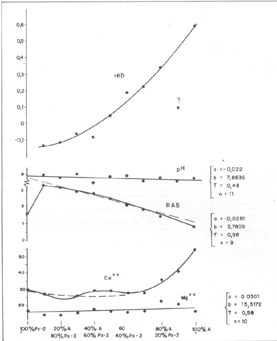
FIGURA 10 - VARIAÇÃO DAS PROPRIEDADES QUÍMICAS DAS MISTURAS DAS AGUAS DO AÇUDE E DO POÇO PZ-2
