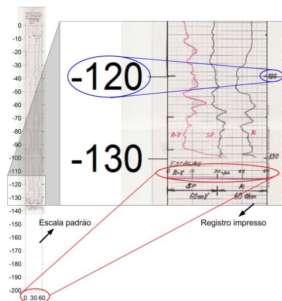
Figura 4 - Exemplificação do método de digitalização dos perfis geofísicos
