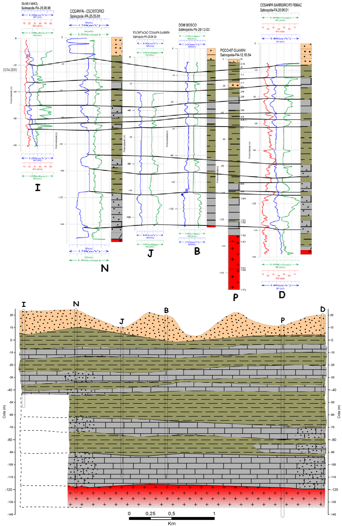
Figura 11 - Seção 4 - Poços I-N-J-B-P-D Figure 11 - Section 4 - Wells I-N-J-B-P-D
