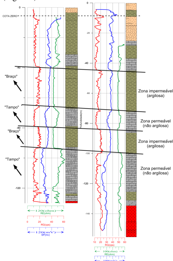
Figura 5 - Representação do Padrão "Violão" Figure 5 - Representation of the "Guitar" model
